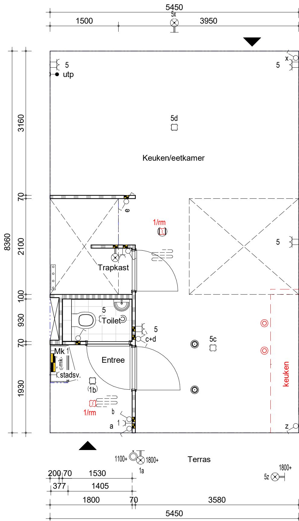
Begane grond
